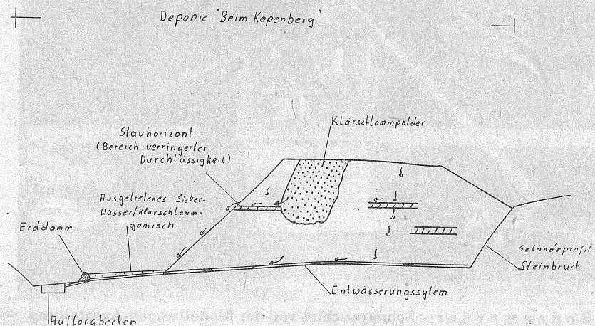
Systemskizze
